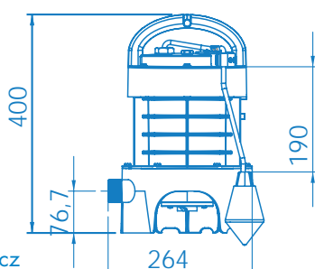
Rozdrabniacz SANIPUMP®
