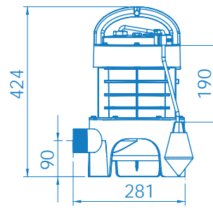
SANIPUMP® Vortex
